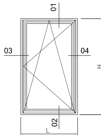
ELEVAÇÃO VISTA EXTERNA S/E
